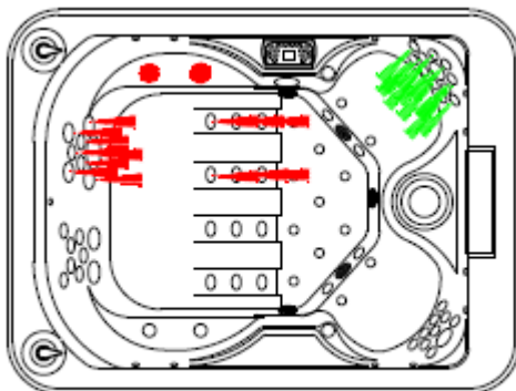
Vodní čerpadlo 1 zapnuto, ovládání trysek (červená pozice, zelená pozice) pomocí ovladače proudu
