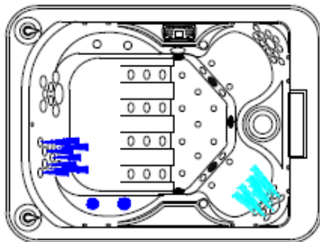
Vodní čerpadlo 2 zapnuto, ovládání trysek (světle modrá pozice, tmavě modrá pozice) pomocí ovladače proudu
